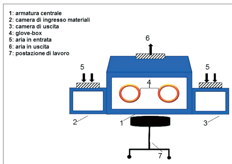
Figura 16 - Isolatore
